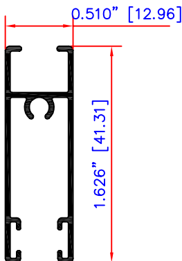
ZOCLO 1519
