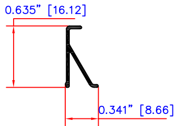
JUNQUILLO 1522
