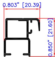
TRAVESAÑO CORREDIZO 1526
