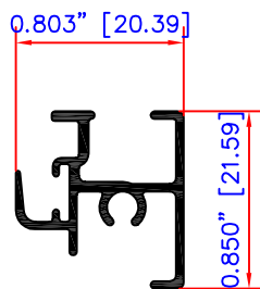
TRAVESAÑO FIJO 1505
